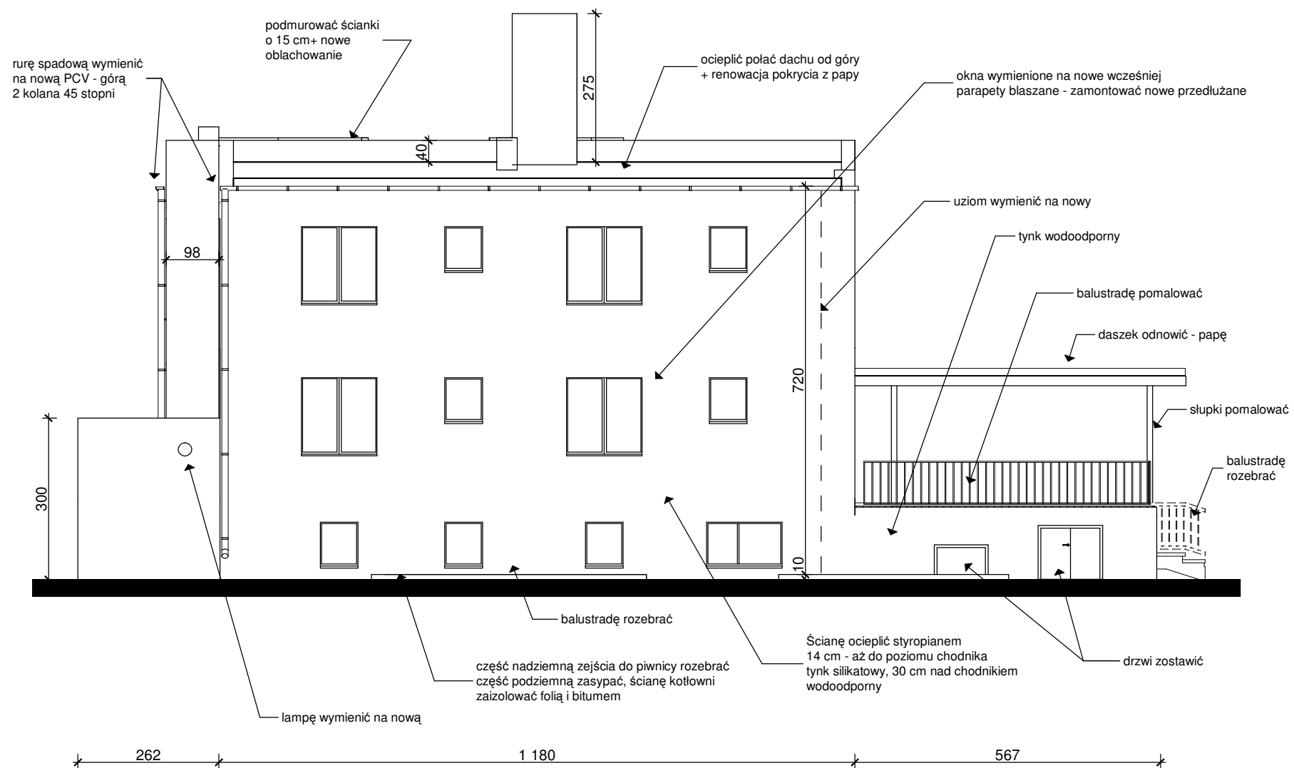
Elewacja boczna zachodnia - termomodernizacja Skala 1:100
