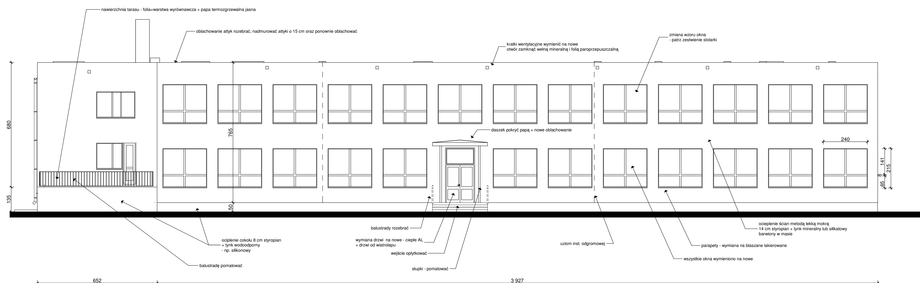
Elewacja frontowa południowa - termomodernizacja Skala 1:100
