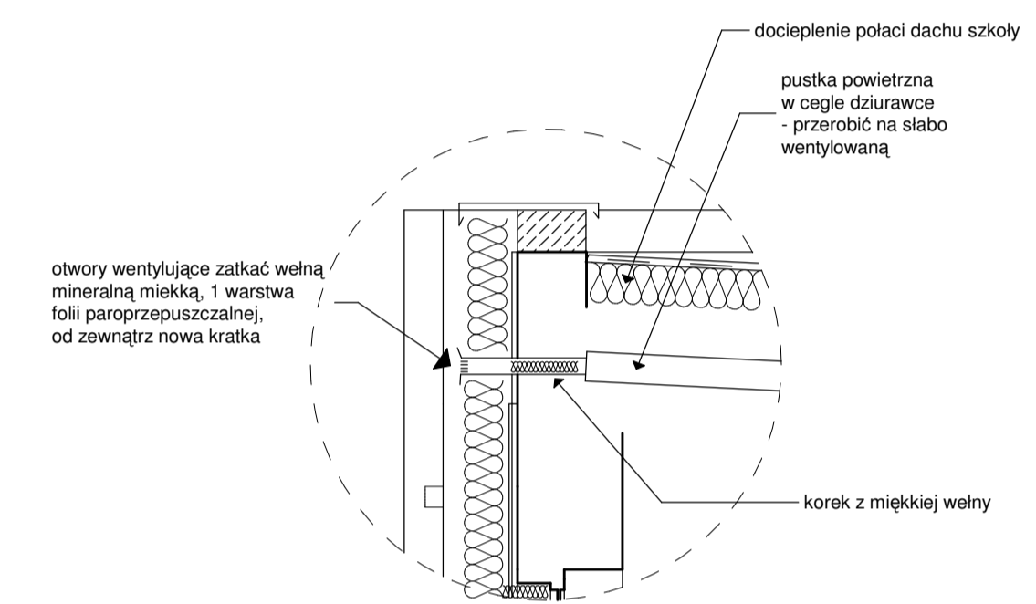
Szczegóły wentylowania pustki powietrznej w dachu
