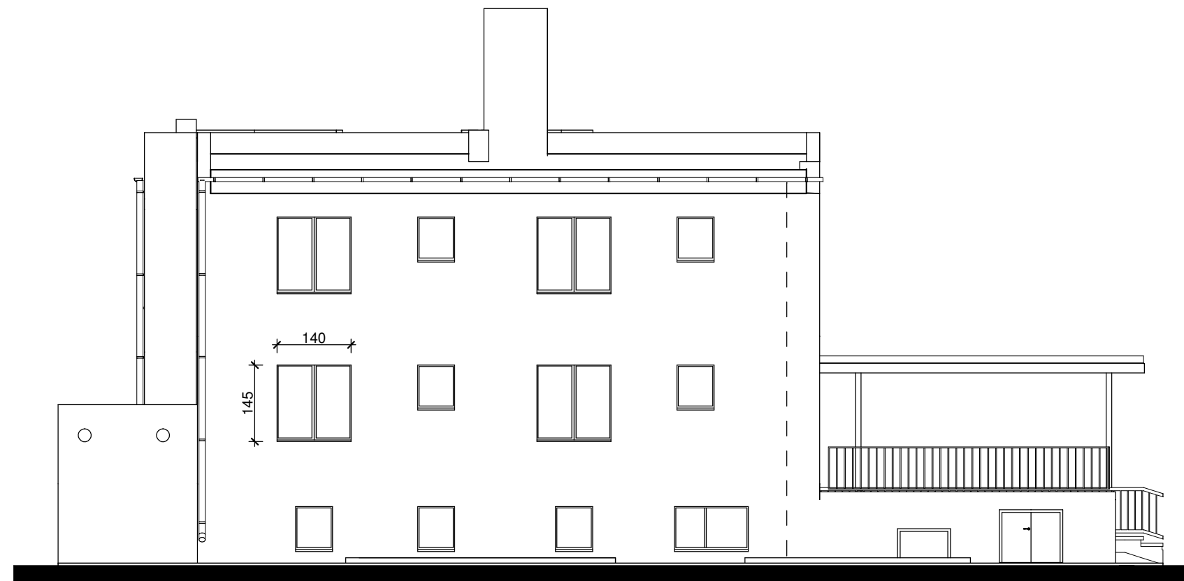
ELEWACJA SZCZYTOWA - zachodnia skala 1:100
