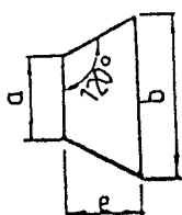
Rysunek I. Kształt płyt betonowych
